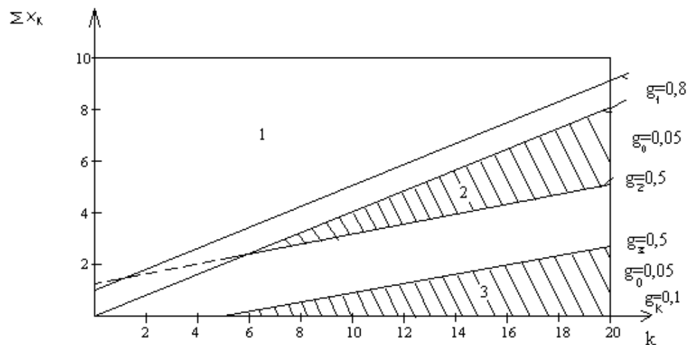
Рис. 1 – Номограма для визначення ефективності продуктів метаноутворення: 1 – незадовільно; 2 – задовільно; 3 – добре.
