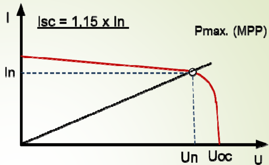
Характеристика I=f(U) модулей PV
