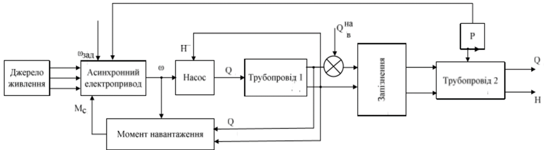
Рис. 1 - Модель насосної станції системи водопостачання
